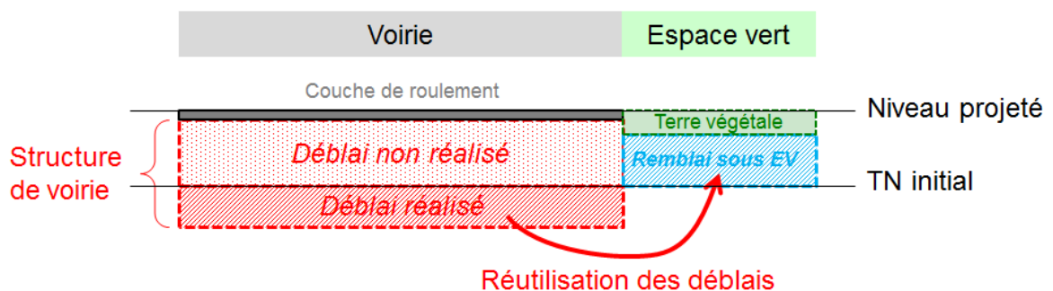
Fig. 23. Schéma de principe du rehaussement et de la réutilisation des déblais
