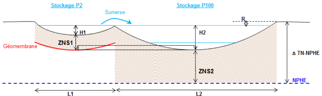
Fig. 32. Profil type d'une noue de stockage et d'infiltration
