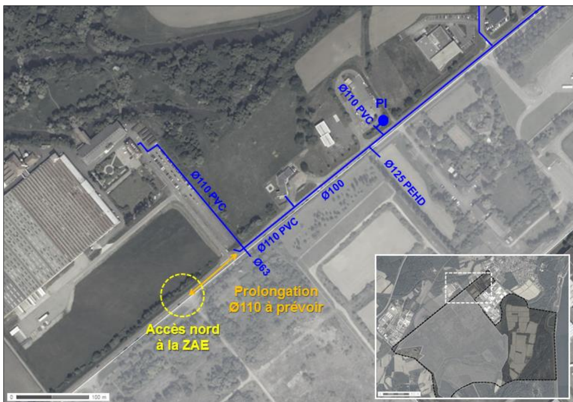
Fig. 28. Plan des réseaux d'eau potable
