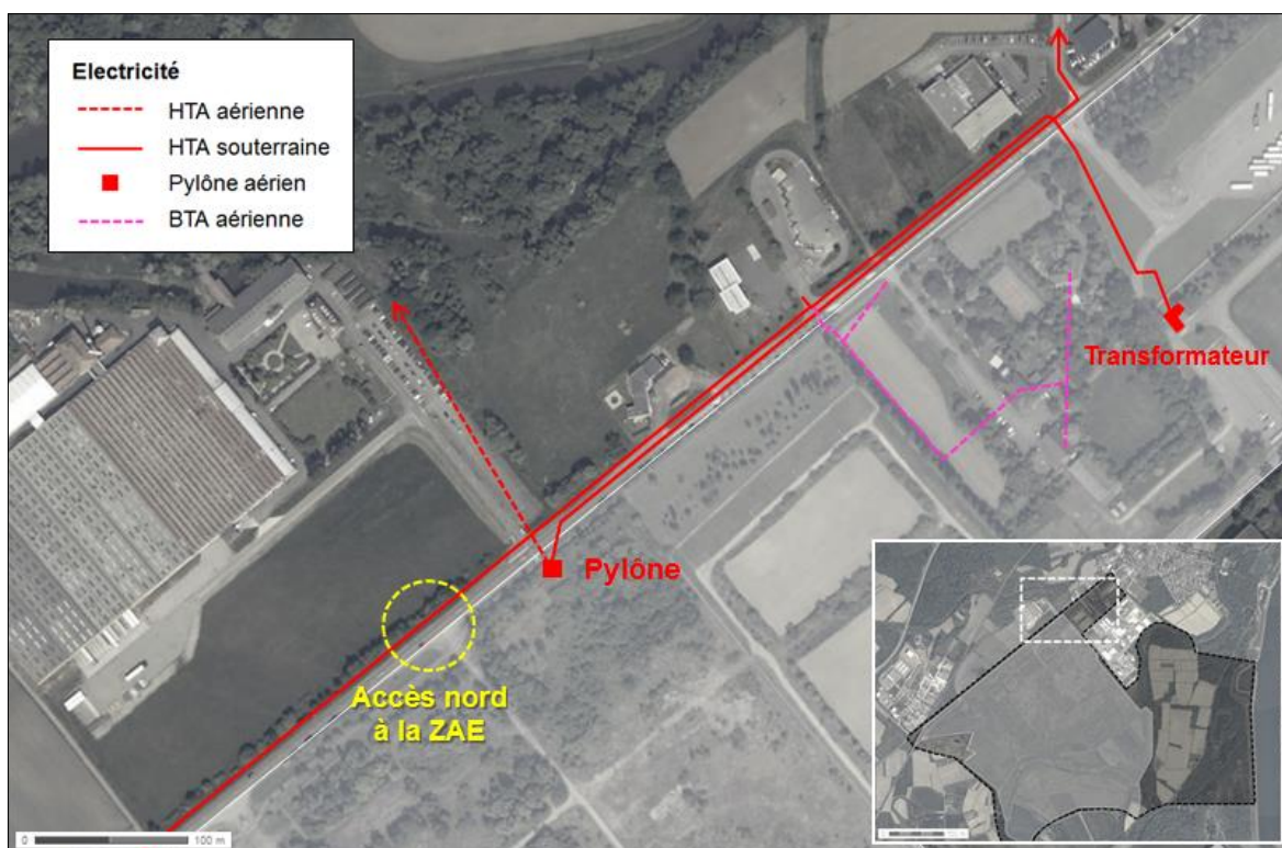
Fig. 26. Plan des réseaux électriques
