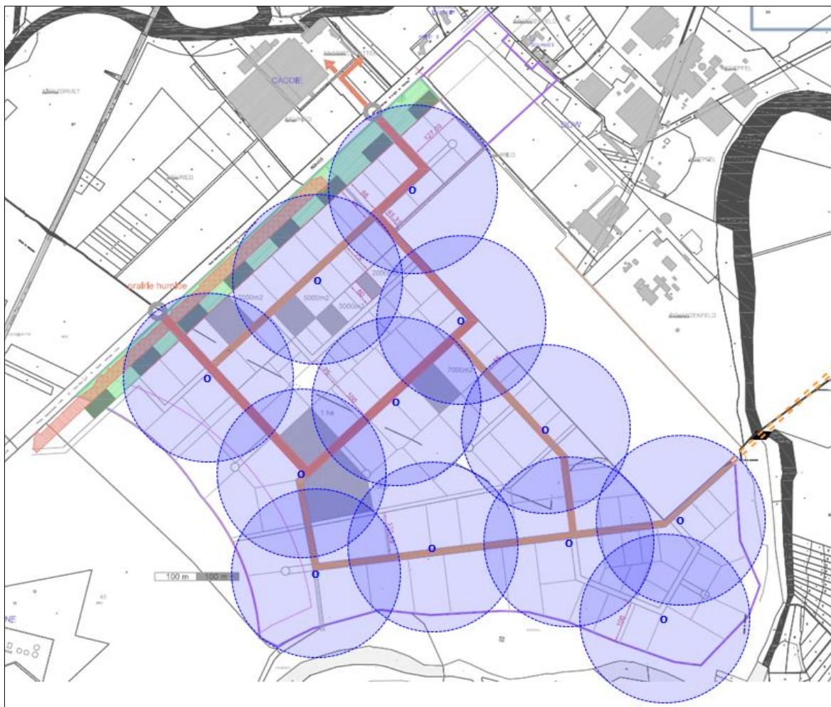
Fig. 29. Localisation et portée de 200 m des puits incendie
