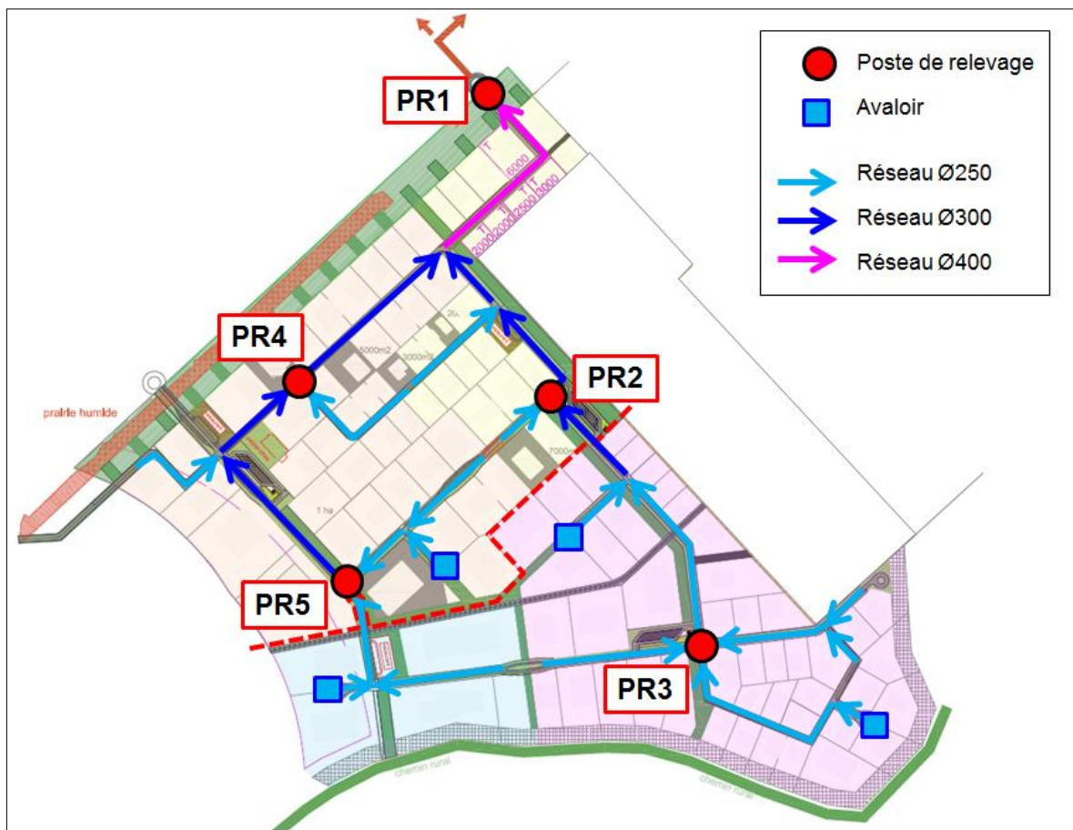
Fig. 30. Plan de réalisation des réseaux d'eaux usées par phase de travaux
