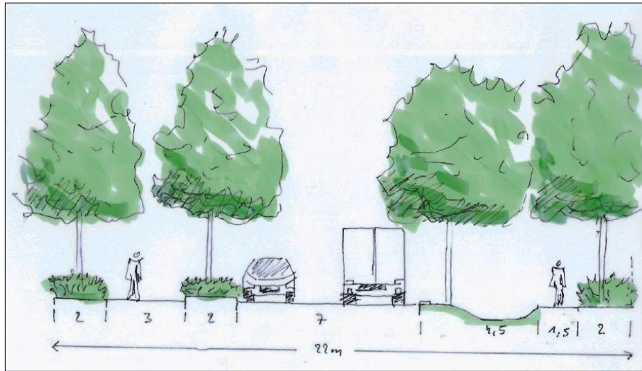
Fig. 49. Voiries primaires – Profil A
