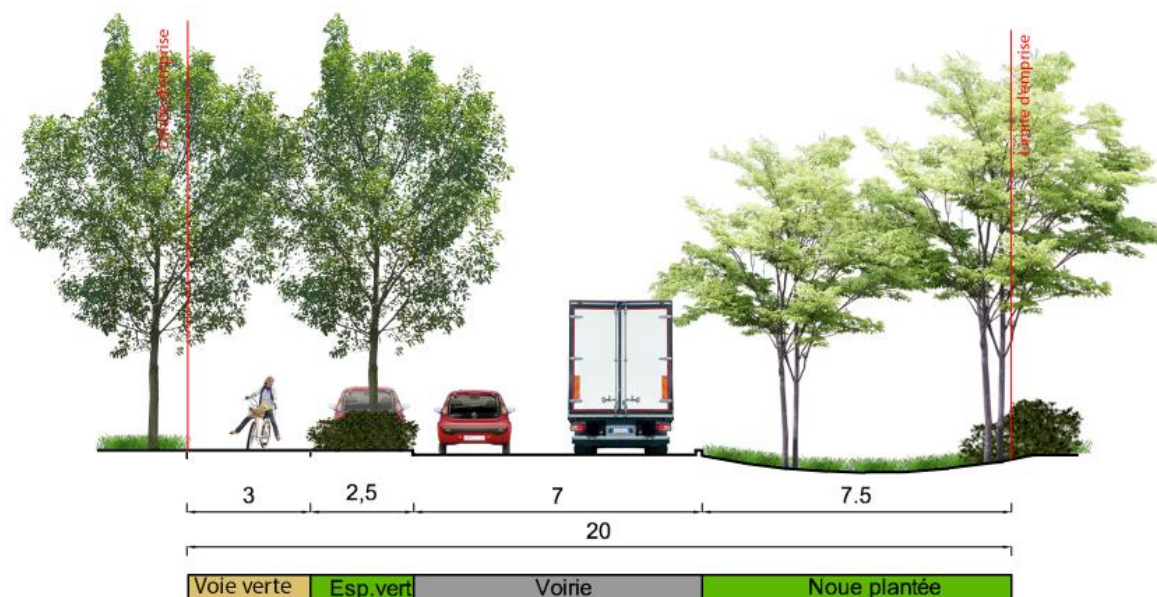
Fig. 11. Profil type des voies primaires
